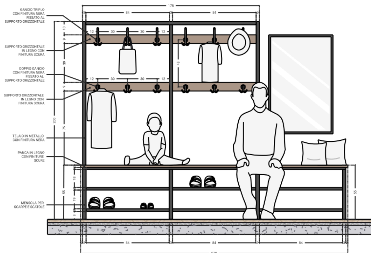
D 1.2 PANCA CON APPENDIABITI - PROSPETTO Scala 1:25
