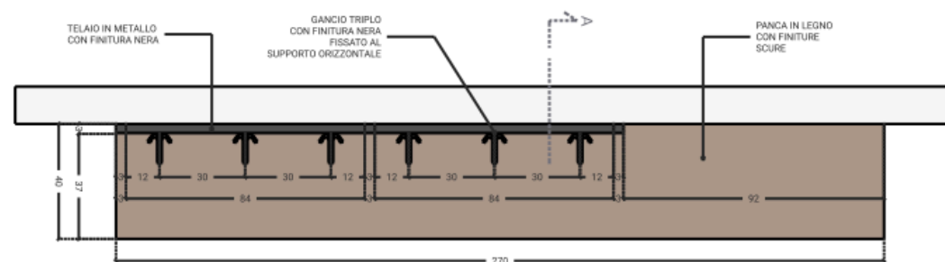
D 1.1 PIANTA DI PANCA CON APPENDIABITI Scala 1:25
