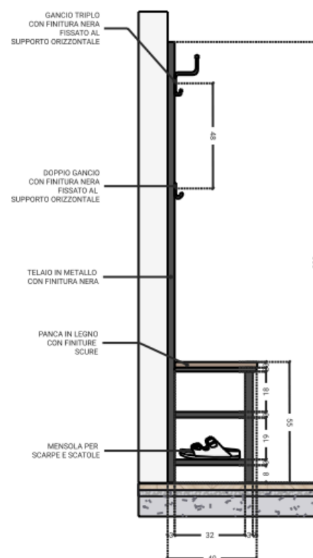
D 1.3 PANCHINA CON APPENDIABITI - SEZIONE A Scala 1:25
